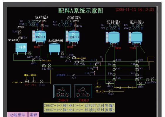
配料流程图
